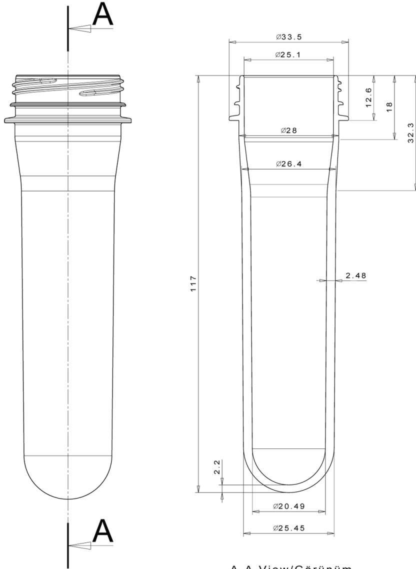
A-A View/Görünüm
